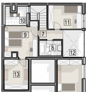
GORNJA ETAŽA
