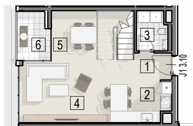
DONJA ETAŽA
